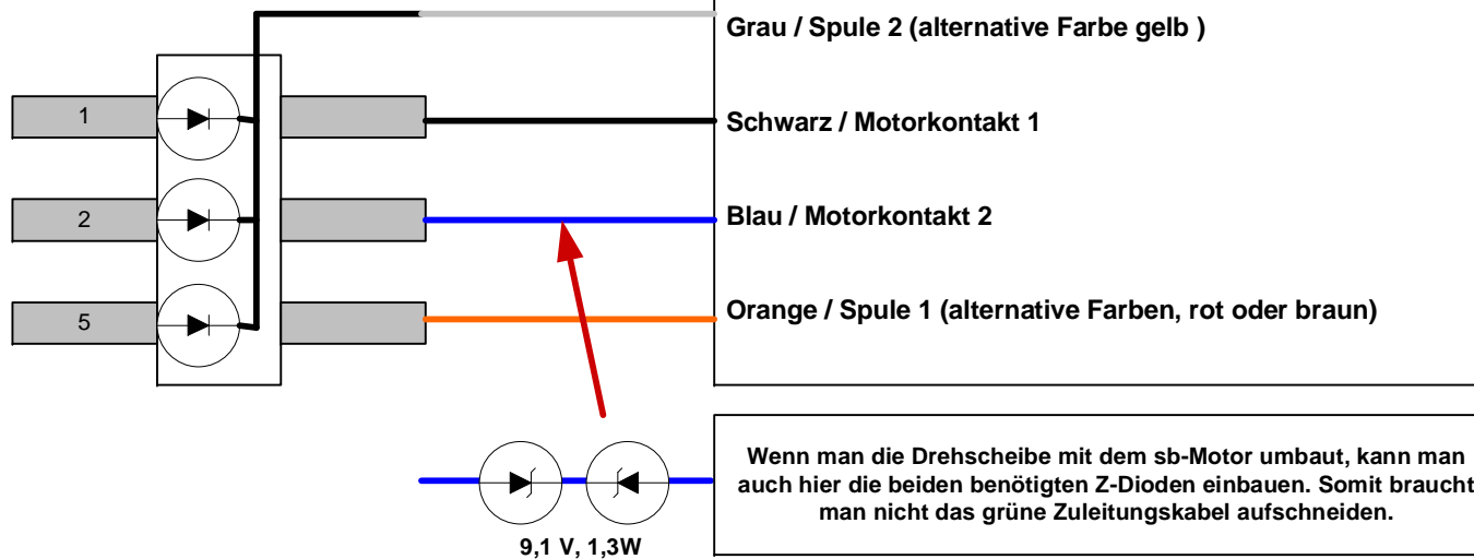
Diodenplatine unter der Bühne 3x 1N 4001
